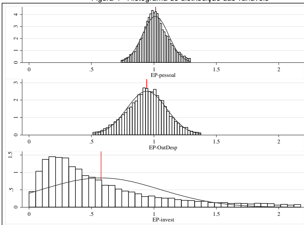
Figura 4 - Histograma de distribuição das variáveis
